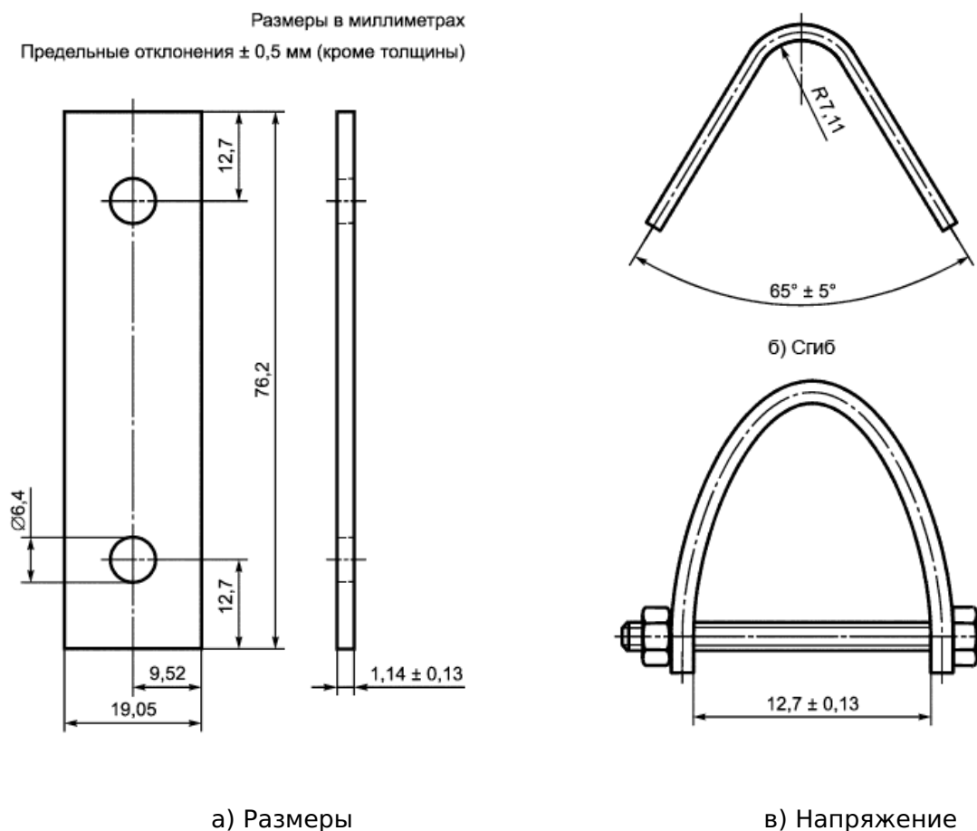
Рисунок 2 - Испытательный образец для испытания на высокотемпературную механическую коррозию титана
